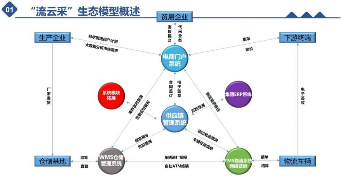
图 11：“流云采”数字供应链平台总体架构
